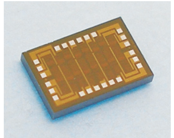
ベアチップ抵抗器 KPC-B Bare Chip Resistor Networks
