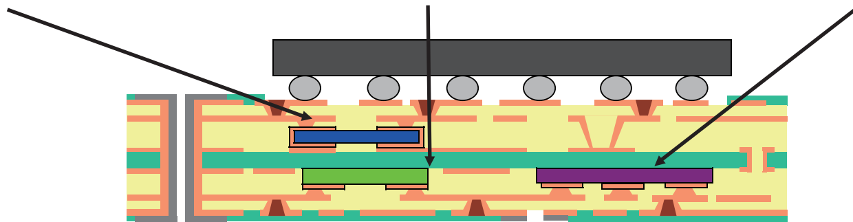
低背厚膜チップ抵抗器 XR73 Low Profile Thick Film Chip Resistors
